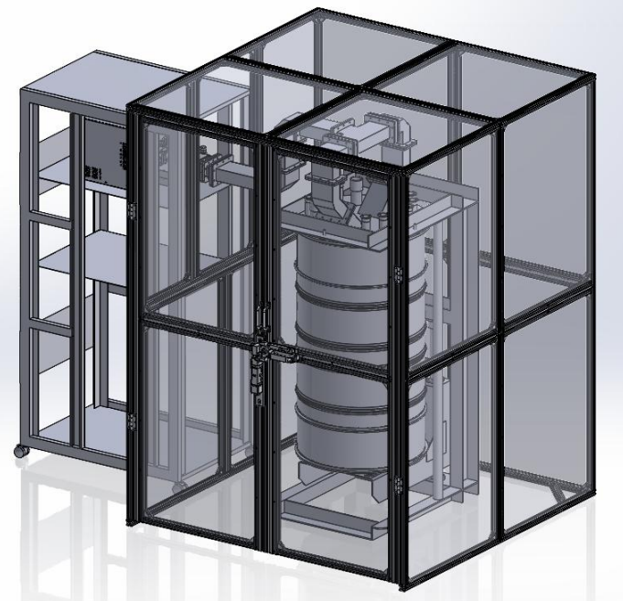
図. 今回開発する試作機イメージ
