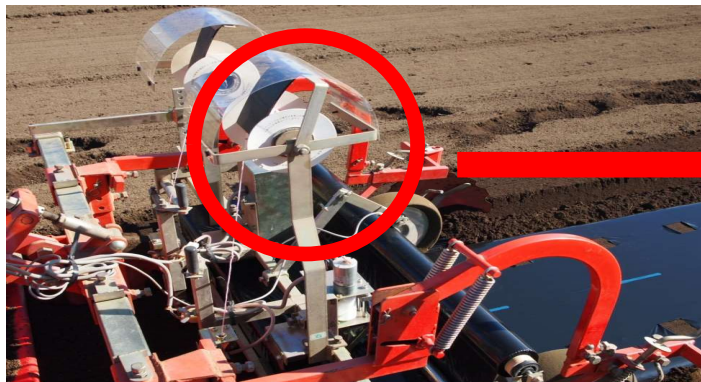
「あけマルくん®(シーダーマシン)」
