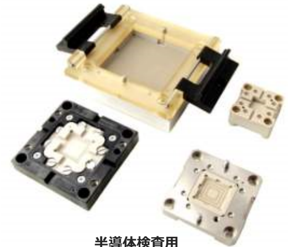
半導体検査用 テストソケット
