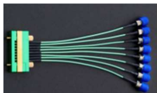
多極同軸コネクタ
