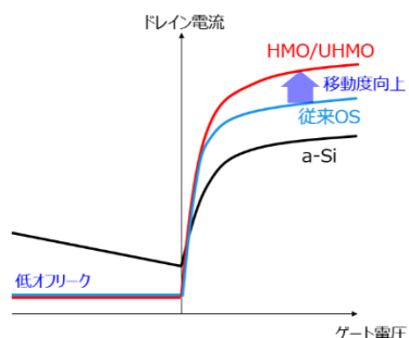
トランジスタ I-V 特性比較図
