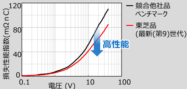
低耐圧MOSFETの優れたON抵抗特性
