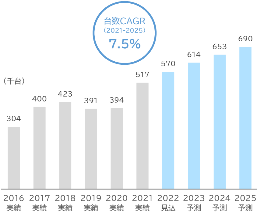
産業用ロボット出荷台数の推移(世界)
