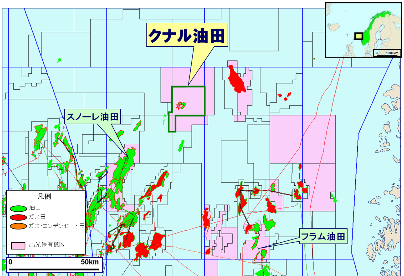
(参考資料) ノルウェー領北海クナル油田位置図
