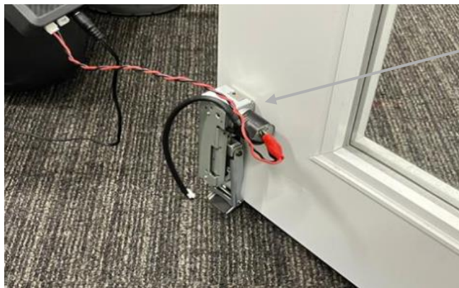
モーターを内蔵した可動式ユニットをドア内部に搭載 (開発中イメージ)
